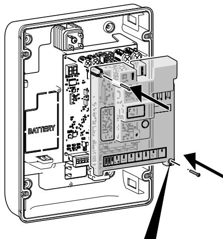
E034 mit Gehäuse
